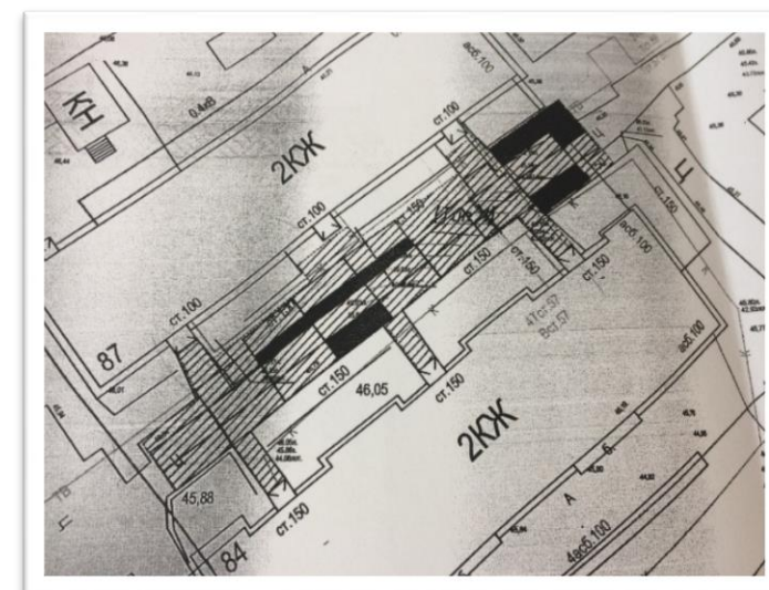
Планировочная схема дворовой территории
